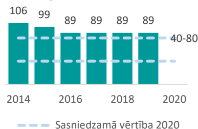
13.2. Vidējais īpatnējā enerģijas patēriņa samazinājums apkurei uz atjaunoto māju dzīvokļu platības kvadrātmetru gadā, kWh/m 2 /gadā
