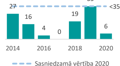
15.11. Gaisa kvalitāte pilsētā: dienu skaits, kad tiek pārsniegta normatīvajos aktos pieļaujamā robežvērtība piesārņojumam ar cietajām daļiņām PM10 Brīvības ielā 73
